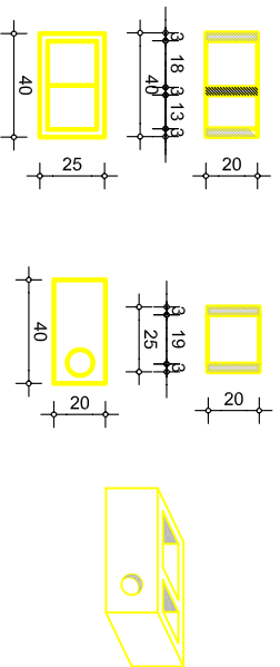
БЕТОШКИ БЛОК "ББ3" CONCRETE BLOCK "BB3"
