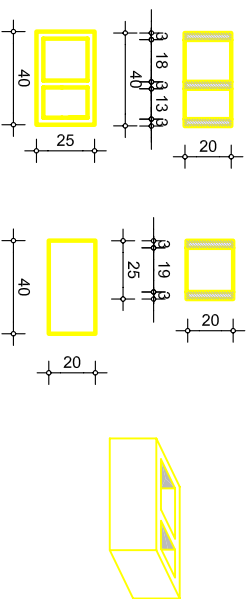
БЕТОШКИ БЛОК "ББ1" CONCRETE BLOCK "BB1"
