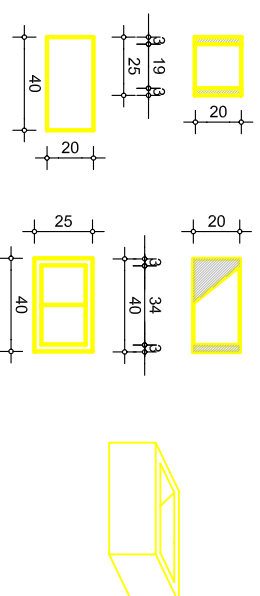
БЕТОШКИ БЛОК "ББ6" CONCRETE BLOCK "BB6"
