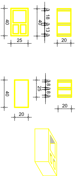
БЕТОШКИ БЛОК "ББ3" CONCRETE BLOCK "BB3"
