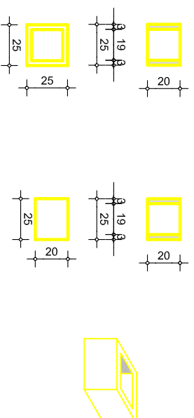
БЕТОШКИ БЛОК "ББ6" CONCRETE BLOCK "BB6"
