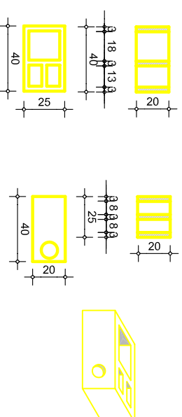
БЕТОШКИ БЛОК "ББ4" CONCRETE BLOCK "BB4"
